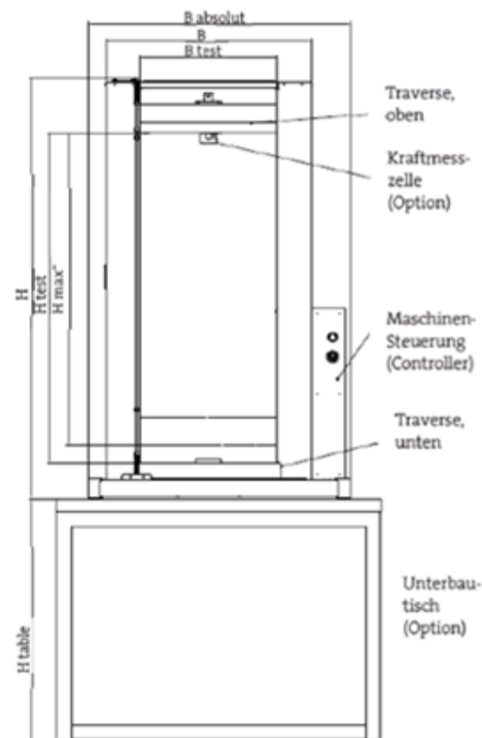
Vorderansicht Prüfmaschine mit Hauptabmessungen
